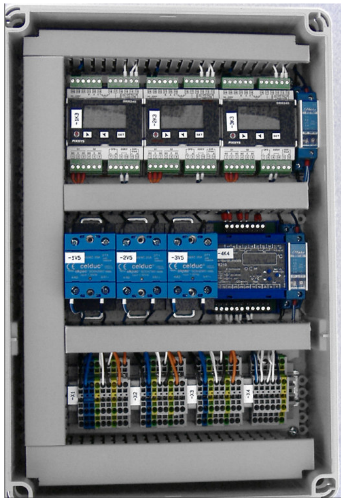
SMB - Standardregler 230 V mit SSR und Kühlkörper bis 25 A-Ausgang -auch für Fronttafeleinbau lieferbar-
